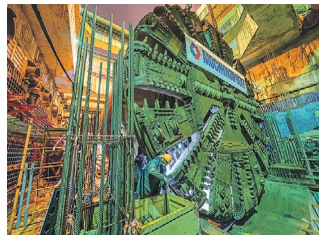
20 января 2020 года. Тоннелепроходческий комплекс «Надежда» в котловане станции «Кунцевская» БКЛ
