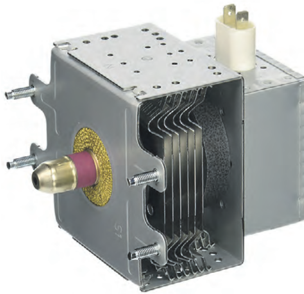
Магнетрон, изобретенный Генрихом Грайнахером, который использовали в работе микроволновой печи
