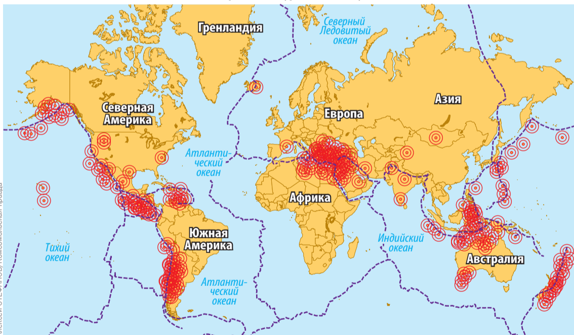
----- Линии разлома между тектоническими плитами ⊙ Сейсмическая активность
