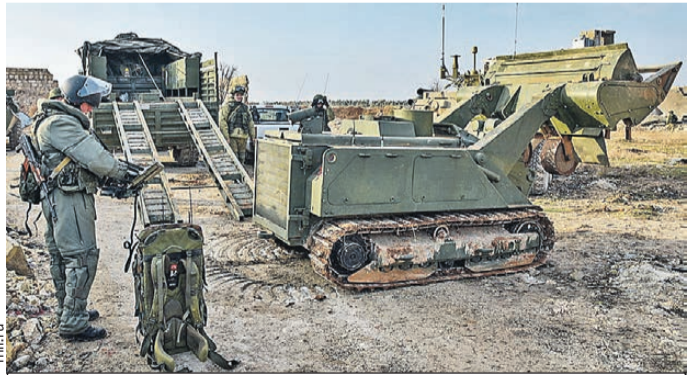
Робот-сапер «Уран-6» на подвиги готов, только ждет команды оператора.
