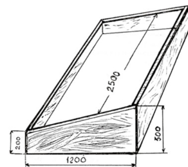
Рис. 2 Деревянный короб для окантовки гряды
